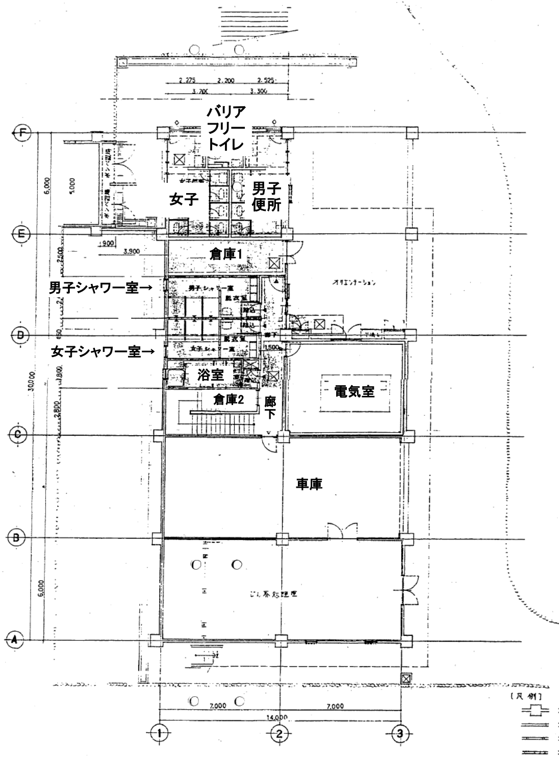
1階平面図
